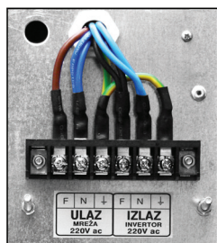
Izgled priključne kutije sa rasporedom klema
